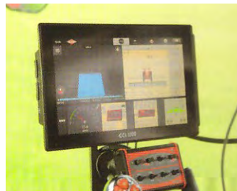
Термінал CCI 1200, встановлений усередині кабіни трактора, використовується для керування причіпним обприскувачем
